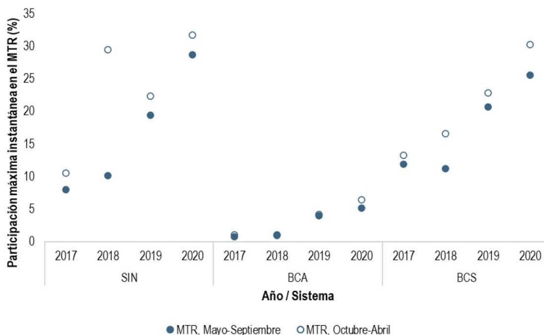
Gráfica 158. Participación de generación instantánea máxima de EO y FV en el MTR, 2017 – 2020
