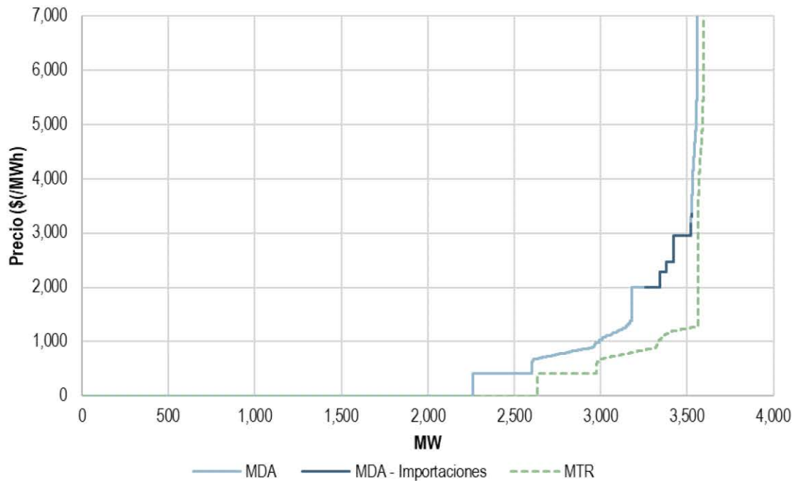
Gráfica 172. Curvas de oferta de asignación en el MDA y MTR del BCA, en la hora 16 del 7 de septiembre de 2020
