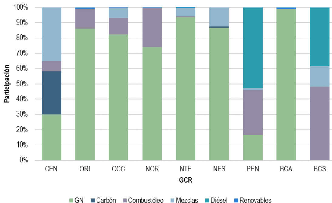
Gráfica 274. Participación de las UCE marginales por tipo de combustible en el MDA por GCR, 2020
