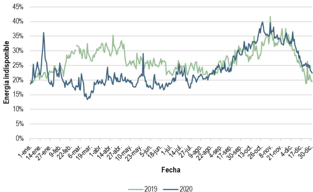
Gráfica 8. Energía indisponible reflejada en las Ofertas de Venta TE en el MDA del SIN, 2019 y 2020
