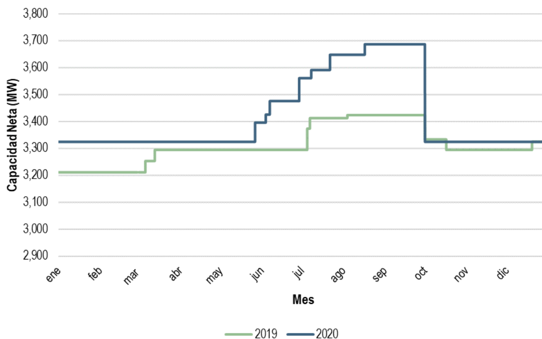
Gráfica 77. Capacidad neta en el BCA, 2019 y 2020
