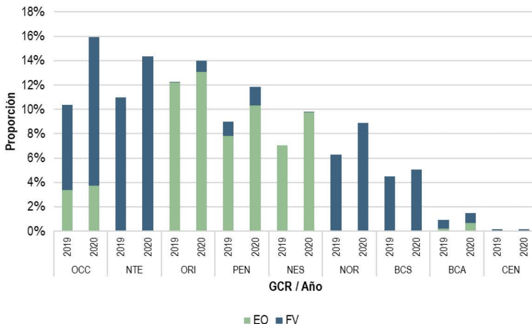
Gráfica 157. Proporción de energía EO y FV generada en Tiempo Real por GCR, 2019 y 2020
