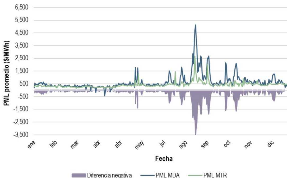
Gráfica 173. PML promedios diarios en el MDA y MTR del BCA, 2020
