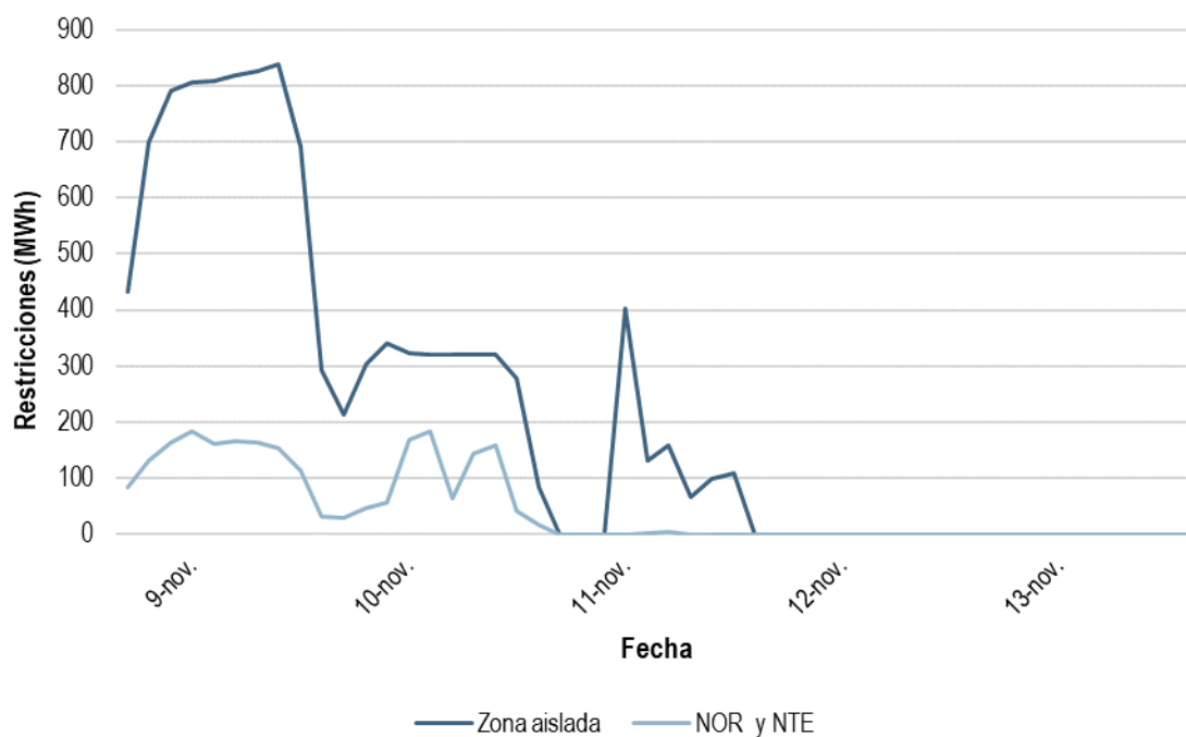
Gráfica 56. Restricciones a la generación RN en el MDA, del 9 al 13 de noviembre de 2020
