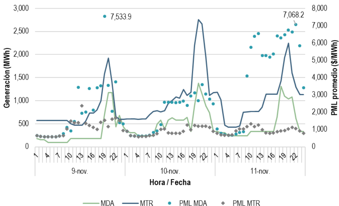
Gráfica 62. Generación HI de la cuenca del río Grijalva y PML promedio en el MDA y MTR, del 9 al 11 de noviembre de 2020
