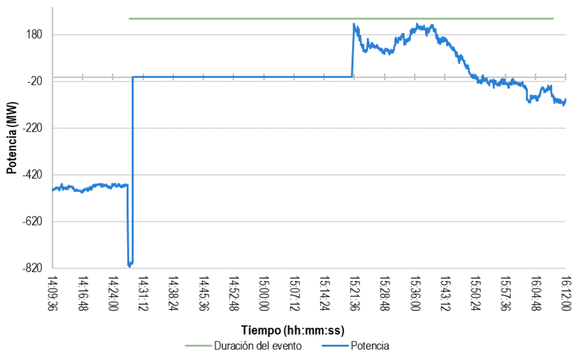
Gráfica 66. Flujo de potencia en la segunda línea de transmisión entre las subestaciones Güémez – Lajas, 28 de diciembre de 2020
