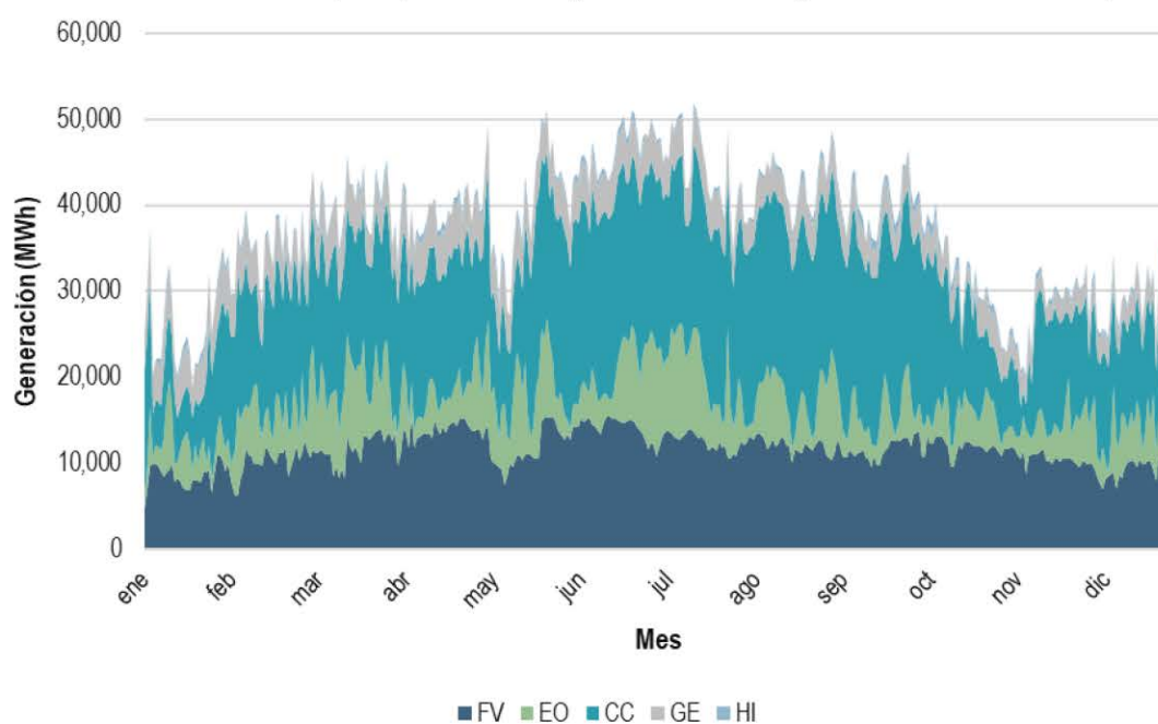
Gráfica 194. Generación por tipo de tecnología de UCE correspondientes a SLP-1/2016, 2020
