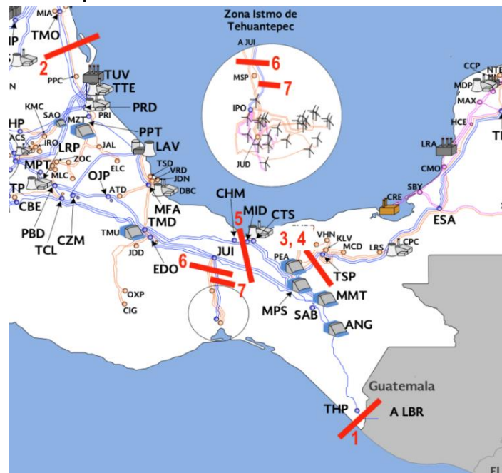
Ilustración 7. Esquema de ubicación de los enlaces de interés de la GCR ORI
