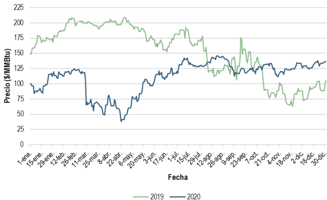
Gráfica 278. Precio promedio diario del combustible empleado para la generación de energía, 2019 y 2020
