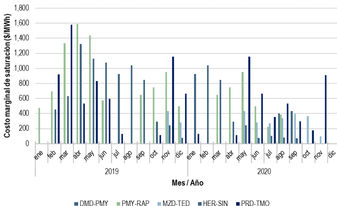
Gráfica 33. Costo marginal de saturación promedio horario por mes en el MDA, 2019 y 2020
