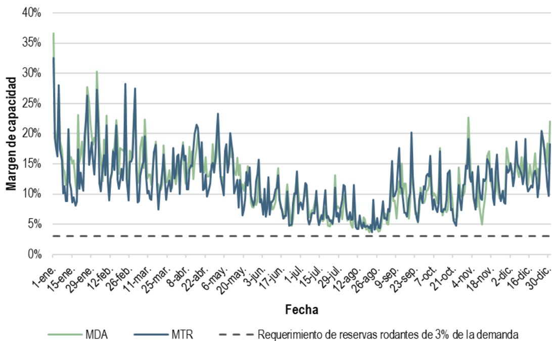
Gráfica 215. Margen de capacidad rodante promedio en el MDA y el MTR del SIN, 2020
