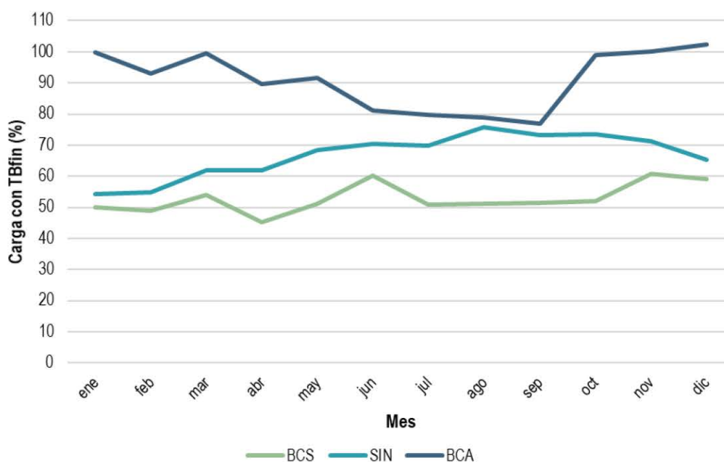
Gráfica 207. Porcentaje de energía que se comercializa en el MDA cubierta por TBFin, 2020
