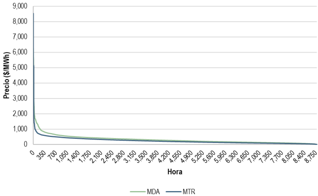
Gráfica 226. Curva de duración de precios de la RREG en el MDA y el MTR del SIN, 2020
