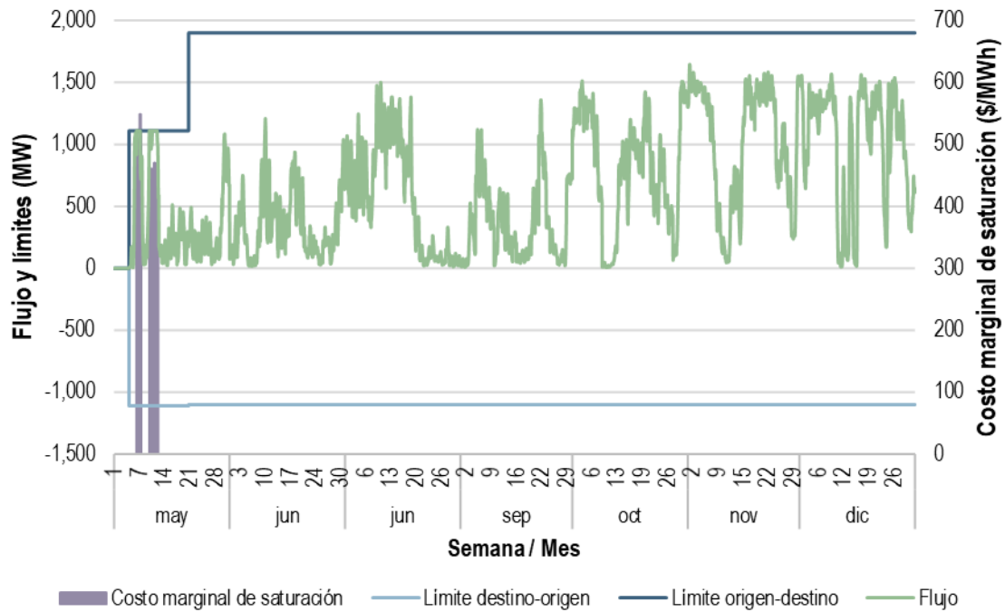
Gráfica 47. Límites de transmisión, flujo y costo marginal de saturación del enlace Ixtepec – Juile en el MDA, mayo a diciembre de 2020
