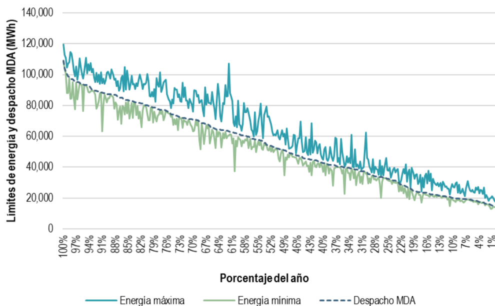
Gráfica 20. Generación Hidroeléctrica de las CE HI en el MDA del SIN, 2020
