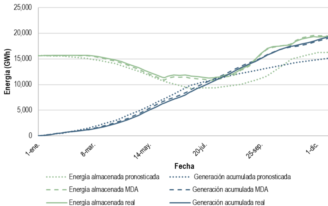
Gráfica 17. Energía almacenada y generación acumulada pronosticada (curva guía), en el MDA y real de las CE HI, 2020
