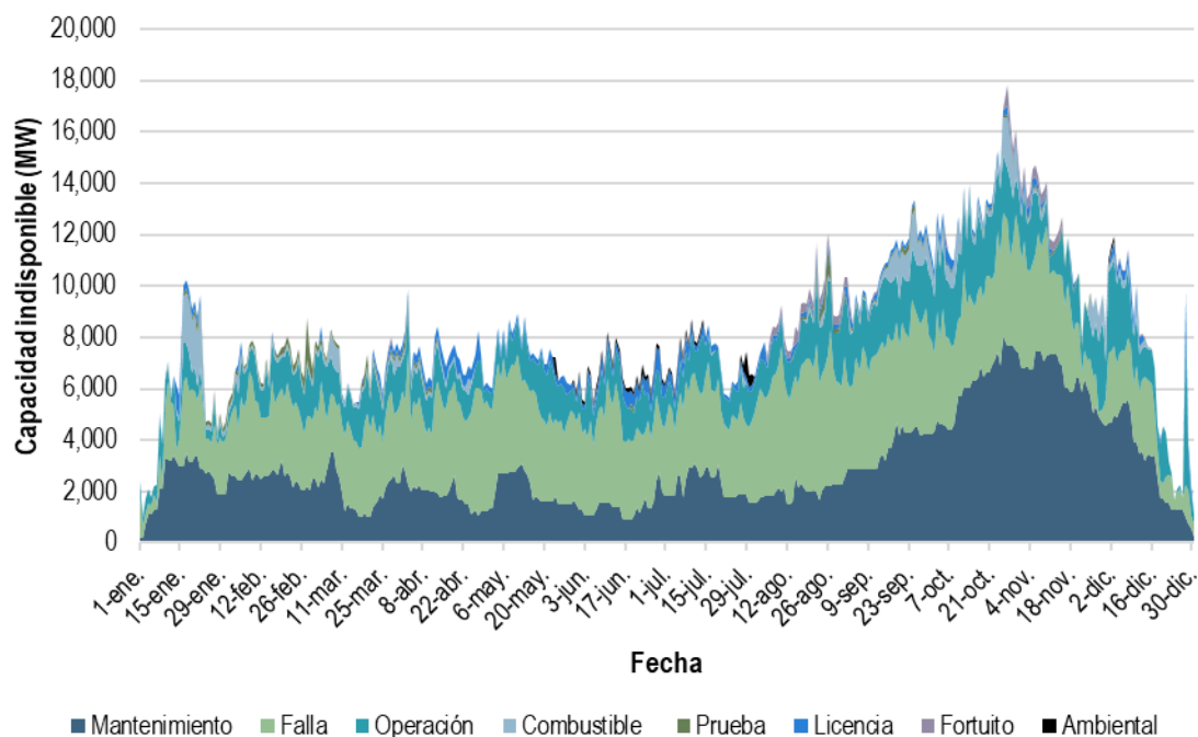
Gráfica 51. Capacidad indisponible en el SIN, 2020
