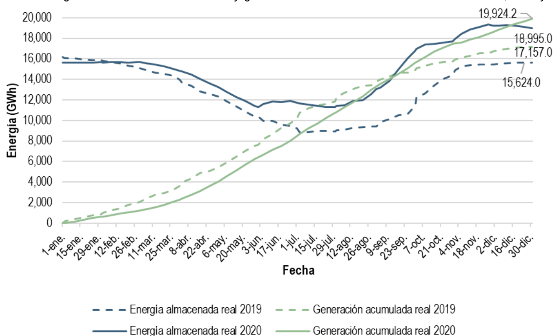
Gráfica 217. Energía hidroeléctrica almacenada y generación hidroeléctrica acumulada en el SIN, 2019 y 2020
