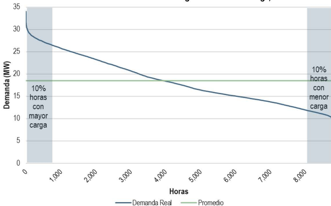
Gráfica 209. Curva de duración de la carga en el Sistema Mulegé, 2020
