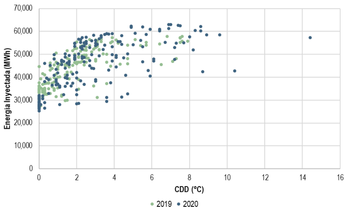
Gráfica 76. Relación entre CDD y la energía inyectada en el BCA, primavera y verano de 2019 y 2020
