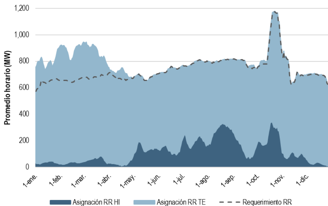
Gráfica 24. Requerimiento y asignación para las RR por Oferta de Venta, 2020
