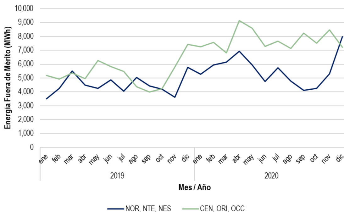
Gráfica 34. EFM promedio mensual en el MDA de las GCR NOR, NTE, NES, CEN, ORI y OCC, 2019 y 2020
