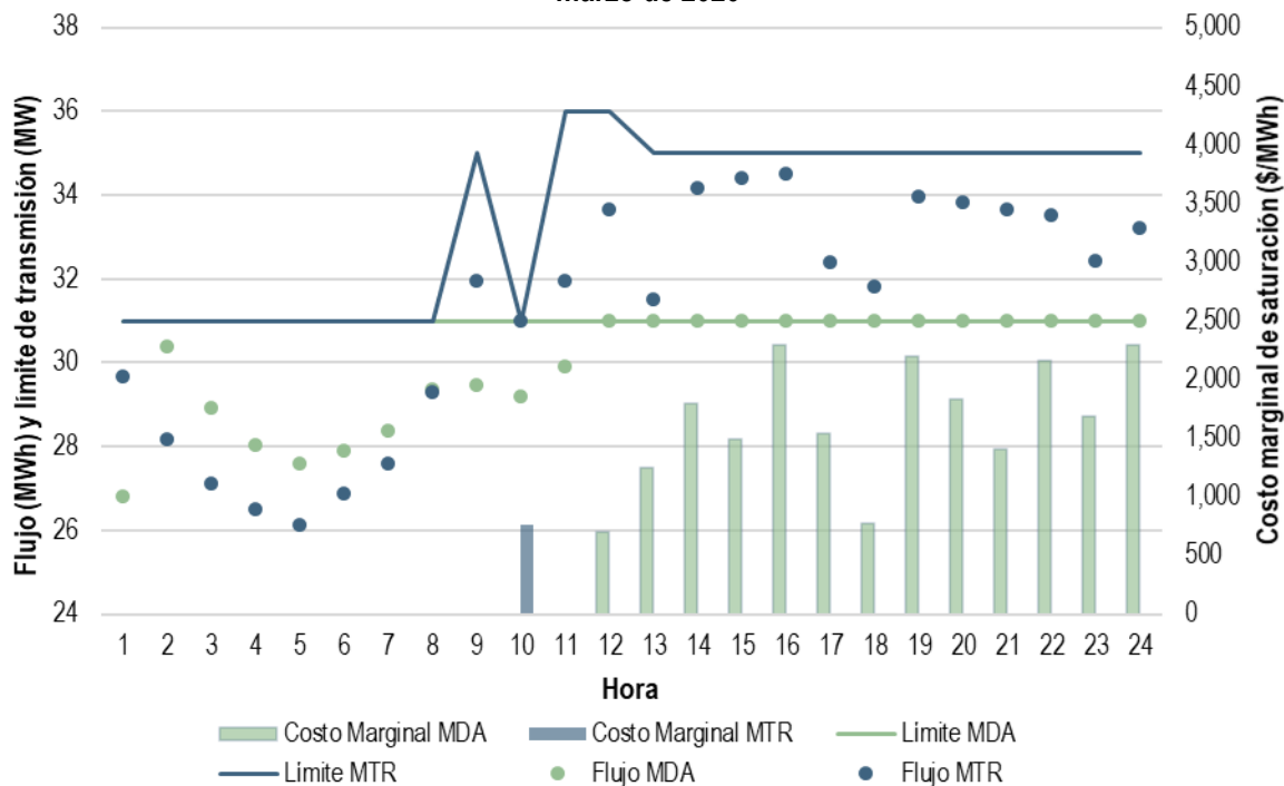
Gráfica 135. Límites de transmisión, flujo y Costo Marginal del enlace Cozumel en el MDA y el MTR, 4 de marzo de 2020
