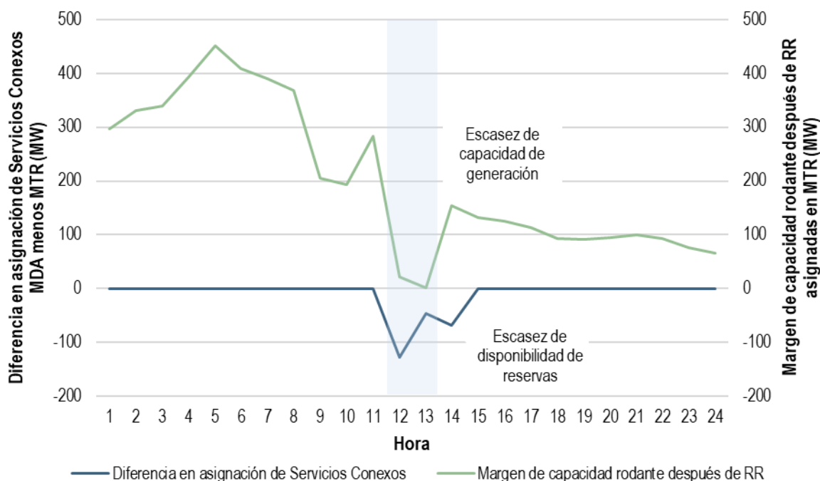
Gráfica 129. Diferencia de reservas asignadas entre el MDA y el MTR, y margen de capacidad rodante después de reservas del MTR del BCA, 26 de octubre de 2020
