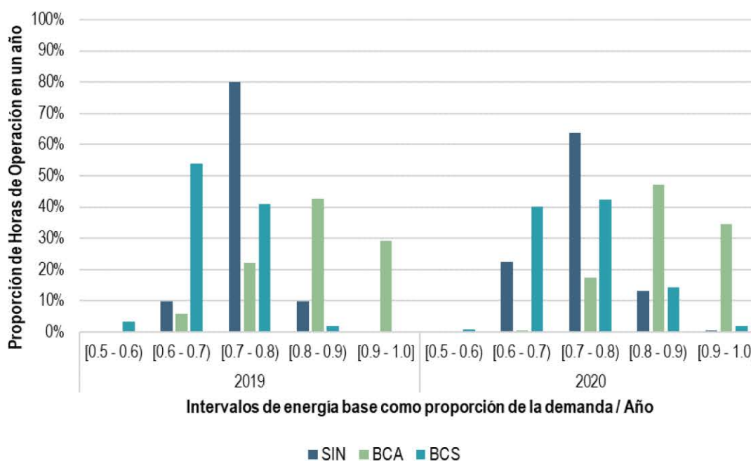
Gráfica 187. Energía base como proporción de la demanda por Sistema Interconectado, 2019 y 2020
