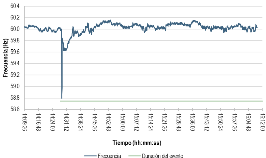
Gráfica 67. Frecuencia del sistema medida en la GCR CEN, 28 de diciembre de 2020
