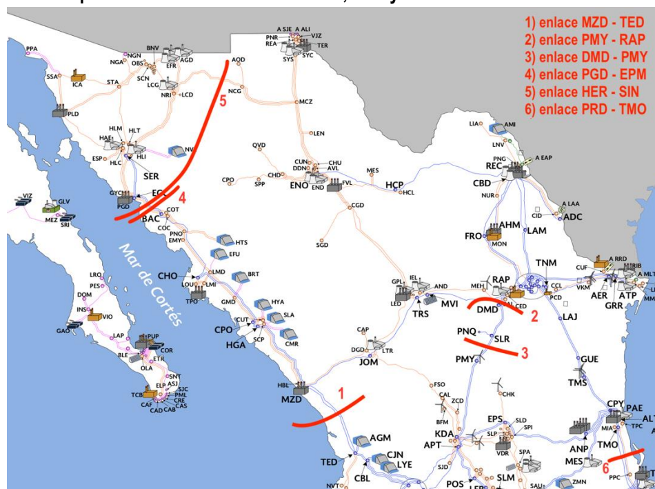
Ilustración 2. Esquema de la RNT de las GCR NOR, NTE y NES e interconexión con el resto del SIN
