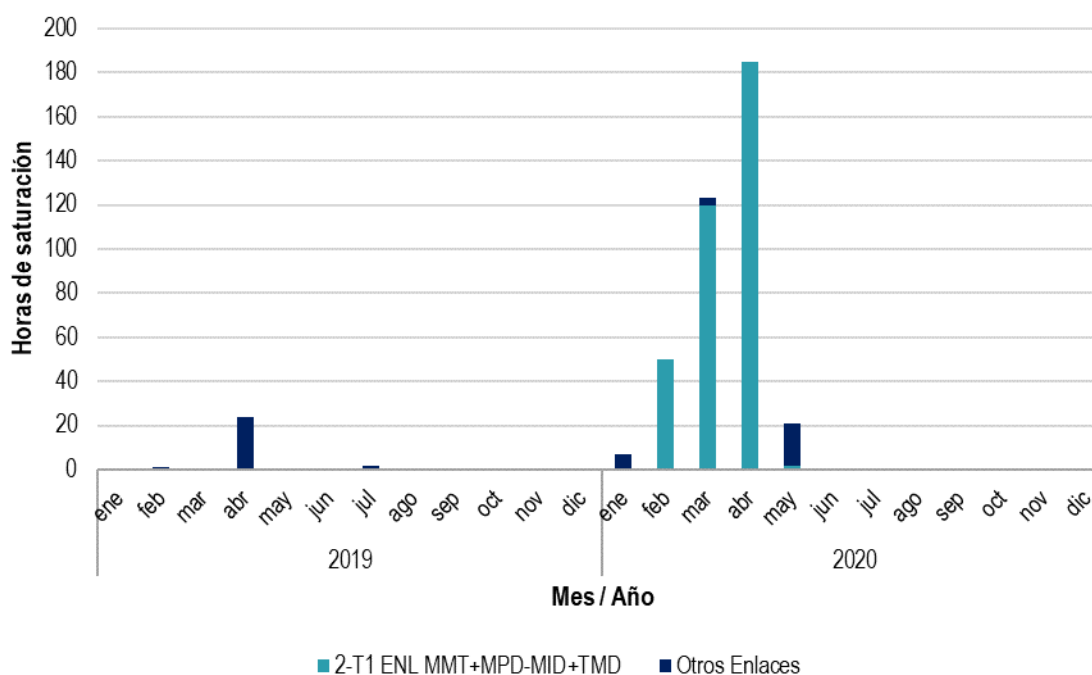
Gráfica 46. Saturación mensual del enlace 2-T1 ENL MMT+MPD-MID+TMD y otros con aplicación temporal, 2019 y 2020
