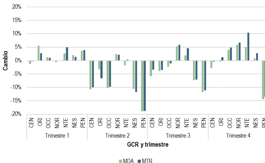
Gráfica 4. Cambio interanual del consumo de energía por trimestre y GCR en el MDA y el MTR del SIN, 2019 y 2020
