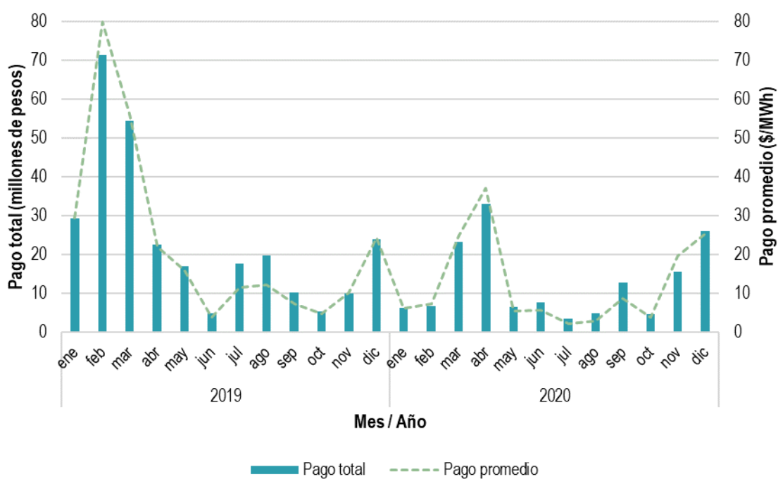
Gráfica 257. Pago total y pago promedio de la GSI en el MDA del BCA, 2019 y 2020
