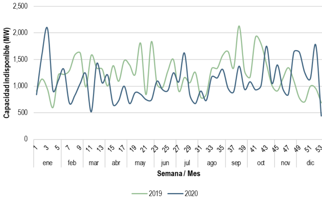
Gráfica 247. Capacidad indisponible por salidas de UCE en el SEN, 2020
