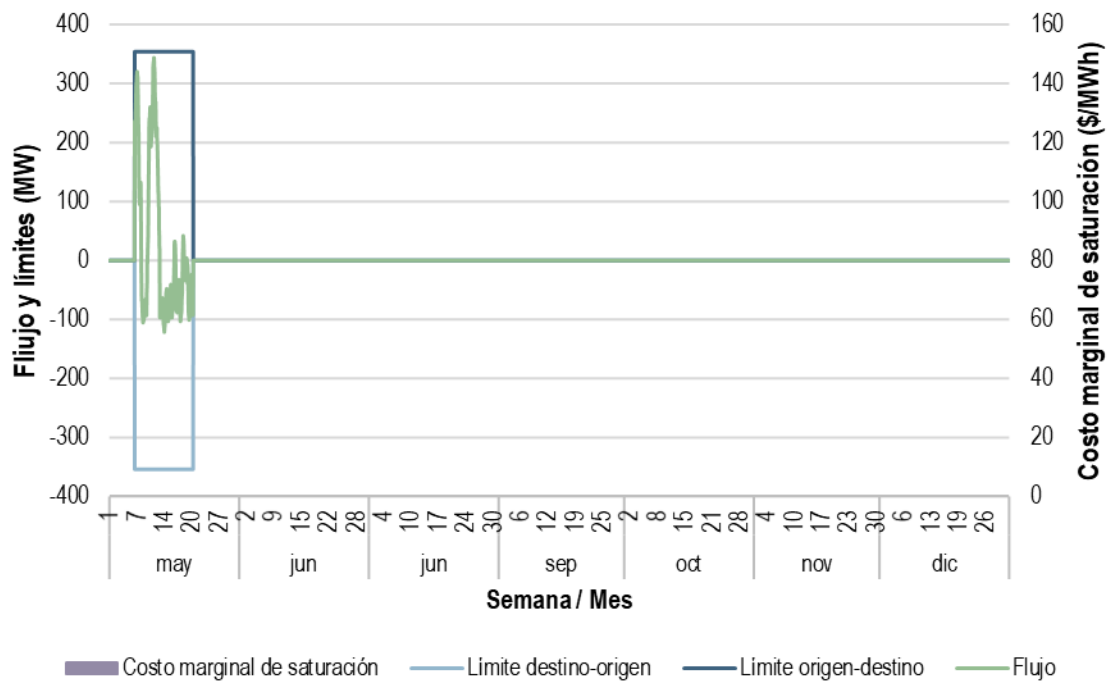
Gráfica 48. Límites de transmisión, flujo y costo marginal de saturación del enlace Juchitán Dos – Juile en el MDA, mayo a diciembre de 2020
