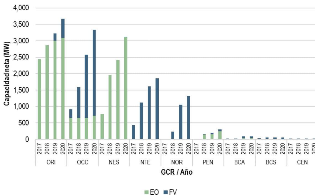
Gráfica 155. Capacidad neta de generación renovable intermitente por GCR, 2017 - 2020
