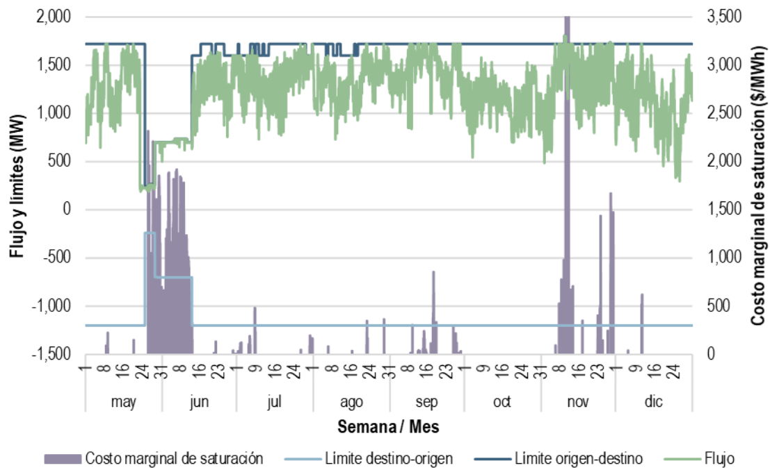
Gráfica 43. Límites de transmisión, flujo y costo marginal de saturación del enlace ORI-NES en el MDA, mayo a diciembre de 2020
