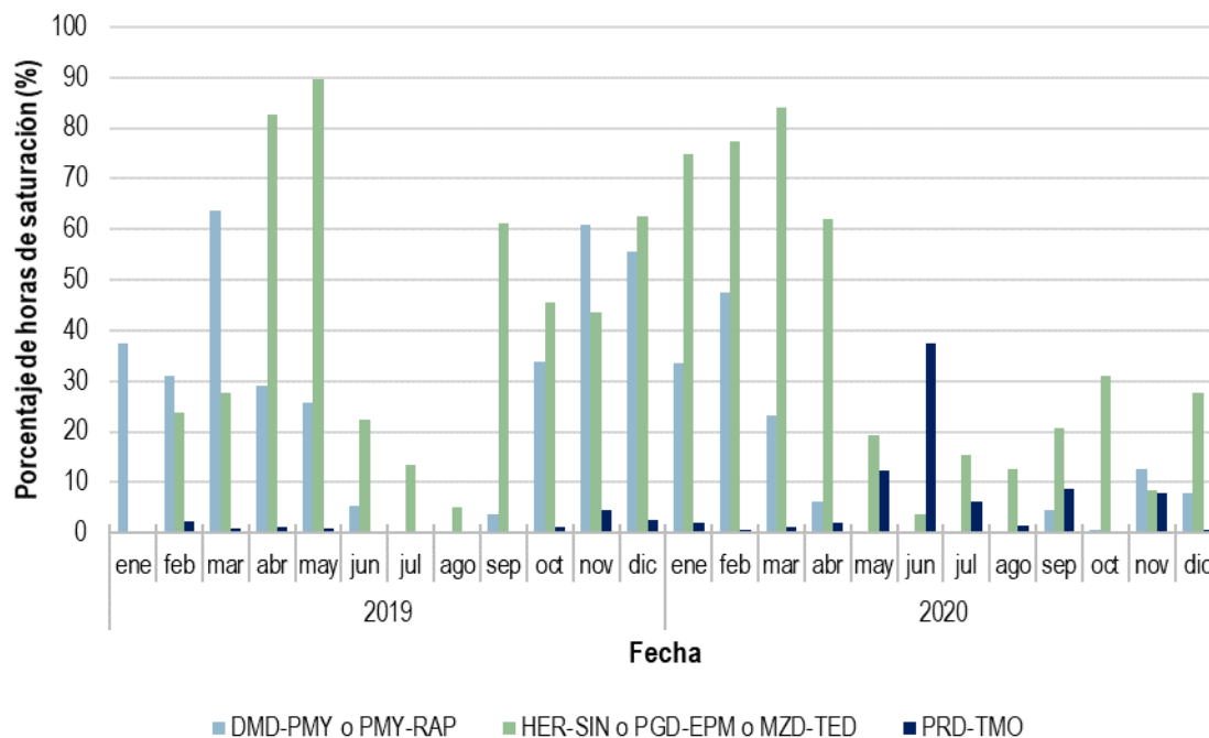
Gráfica 29. Saturación de los enlaces MZD-TED, DMD-PMY o PMY-RAP, HER-SIN o PGD-EPM y PRD-TMO en el MDA, 2019 y 2020
