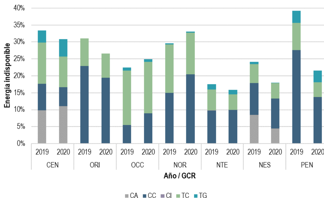
Gráfica 9. Energía indisponible reflejada en las Ofertas de Venta TE en el MDA por tipo de tecnología y GCR del SIN, 2019 y 2020
