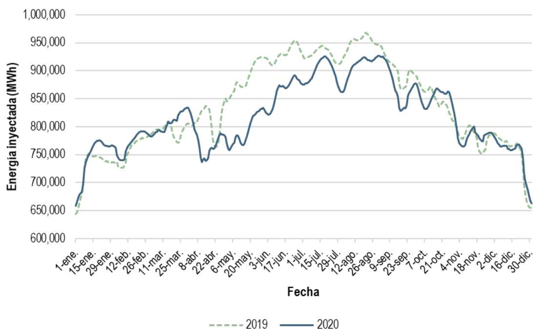
Gráfica 3. Energía inyectada promedio diaria en el MDA del SIN, 2019 y 2020
