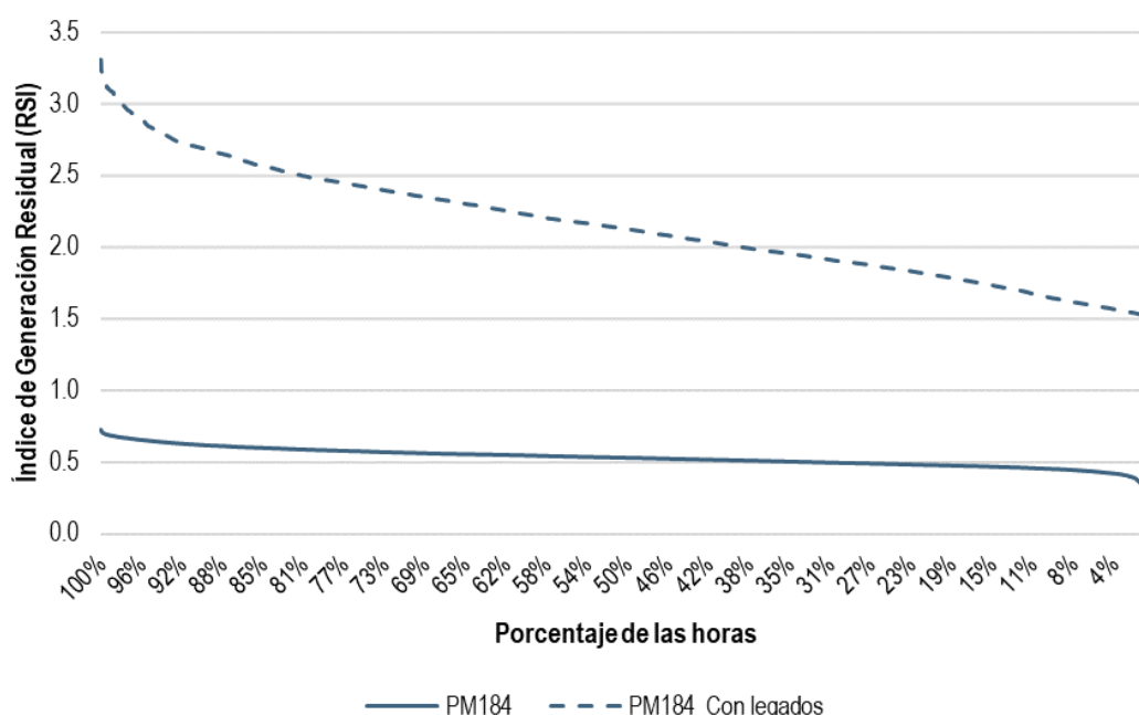
Gráfica 120. BCA: RSI con y sin CLSB, 2020
