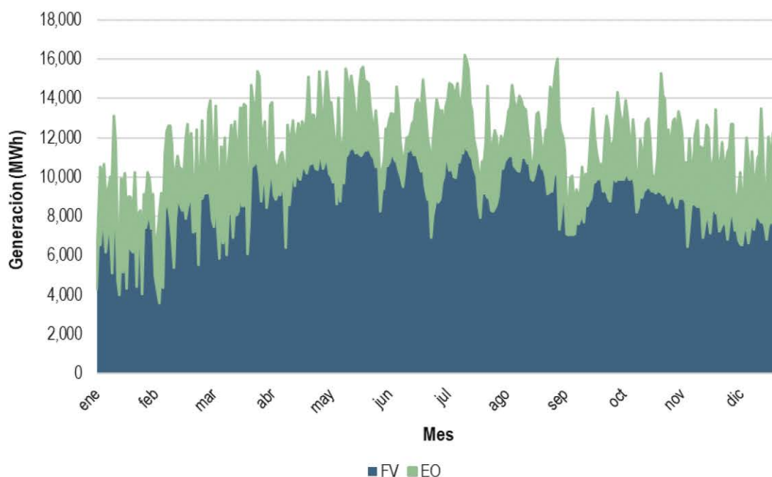
Gráfica 193. Generación por tipo de tecnología de UCE correspondientes a SLP-1/2015, 2020
