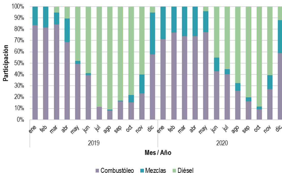
Gráfica 102. Participación de las UCE marginales por tipo de combustible en el MDA del BCS, 2019 y 2020
