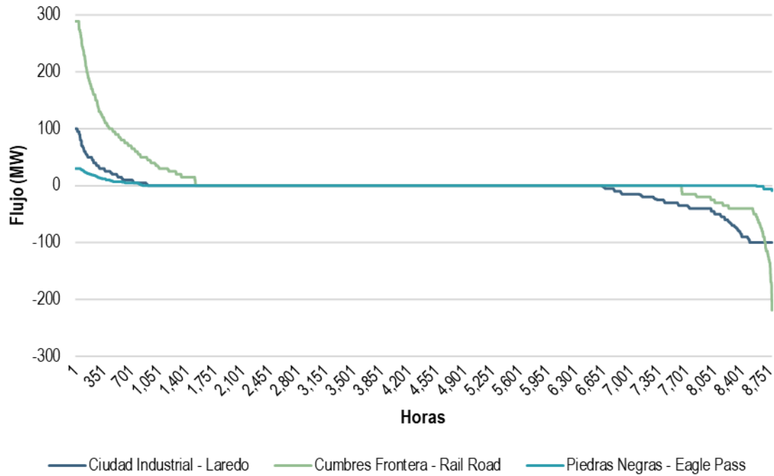
Gráfica 229. Curva de duración de flujos internacionales de energía en los Enlaces de Interconexión del SIN con ERCOT, 2020
