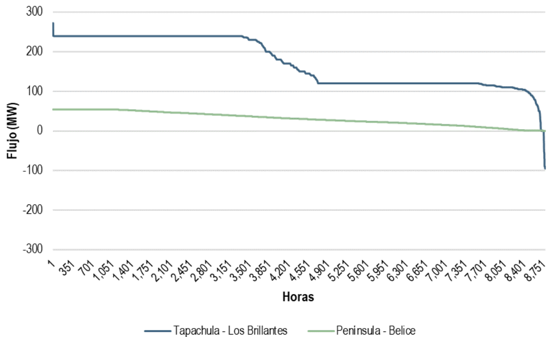
Gráfica 230. Curva de duración de flujos internacionales de energía en los Enlaces de Interconexión del SIN con Guatemala y Belice, 2020
