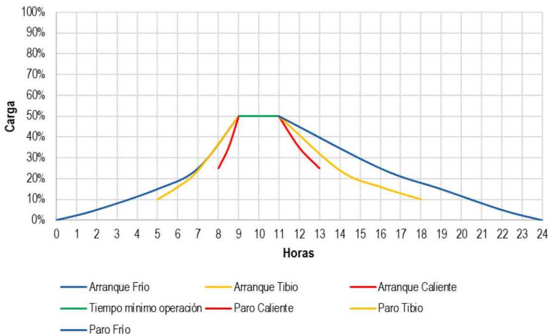
Gráfica 192. Ciclo mínimo de operación de una UCE de Oferta de Venta TE
