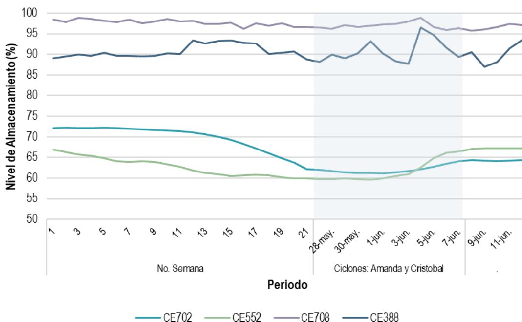
Gráfica 19. Volumen de almacenamiento de las CE con Oferta de Venta HI pertenecientes a la cuenca del río Grijalva, enero a junio de 2020
