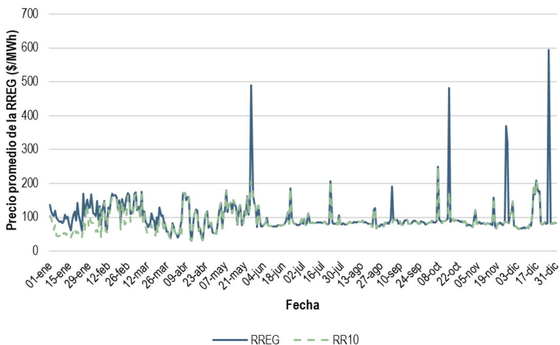
Gráfica 114. Precio promedio diario de la RREG y la RR10 en el MDA del BCS, 2020
