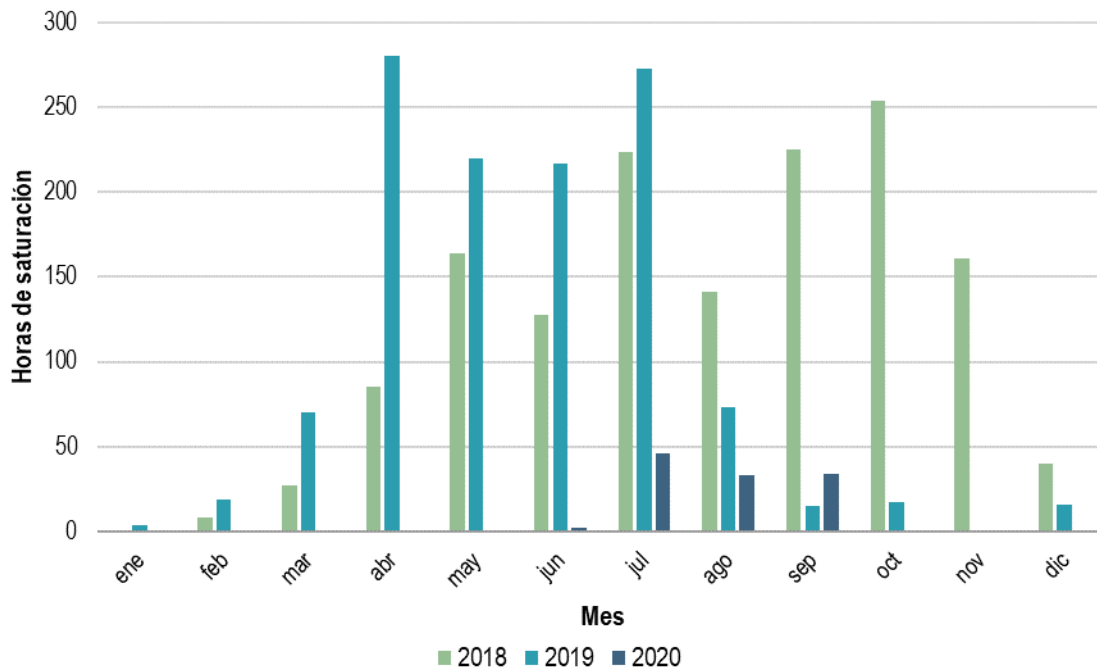
Gráfica 36. Saturación del enlace ESA en el MDA que limita el intercambio entre las GCR PEN y ORI, 2018, 2019 y 2020
