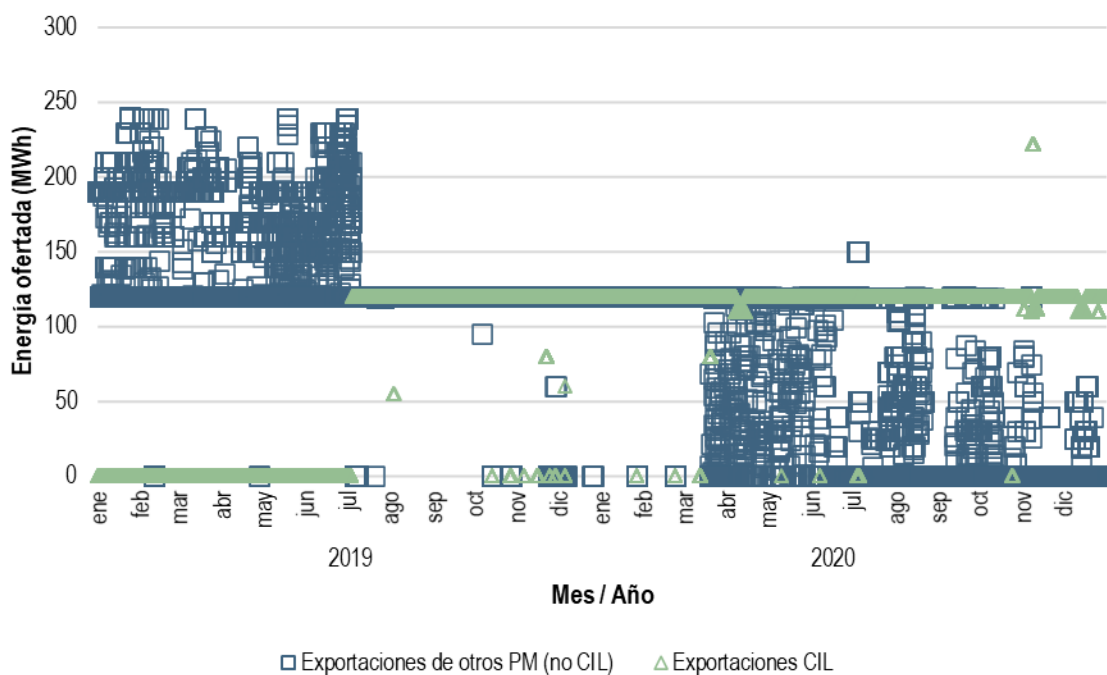
Gráfica 39. Exportaciones de energía en el MDA y nodo 09LBR-230, de 2019 y 2020
