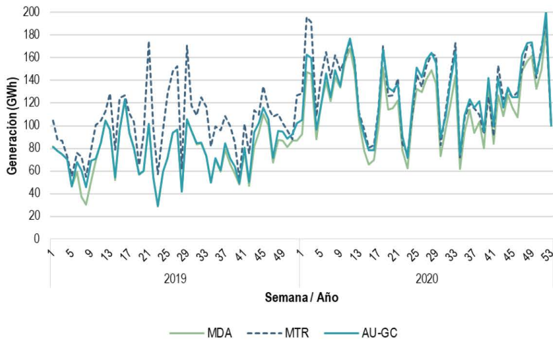
Gráfica 161. Suma semanal de generación EO (Oferta de Venta RN) en el MDA, AU-GC y MTR, 2019 y 2020
