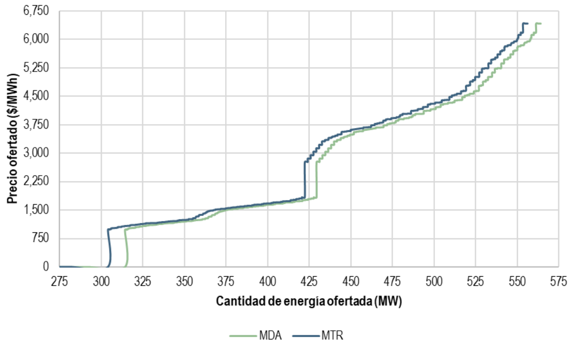
Gráfica 239. Curvas de oferta promedio de energía en el MDA y el MTR del BCS en la hora 20, 2020
