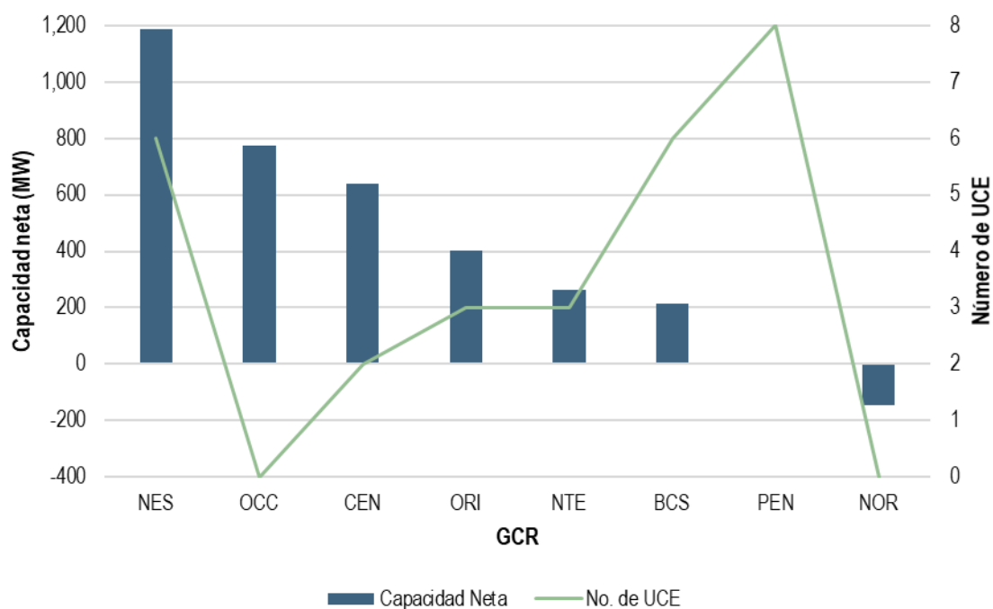
Gráfica 122. Cambio en la capacidad neta por altas y bajas y número de UCE del SEN por GCR, 2020
