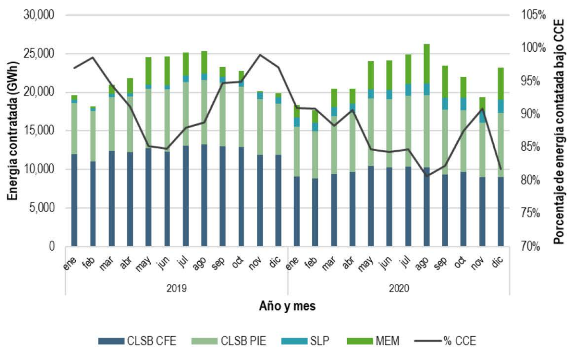
Gráfica 205. Energía eléctrica contratada estimada para el Suministro Básico (CLSB)
