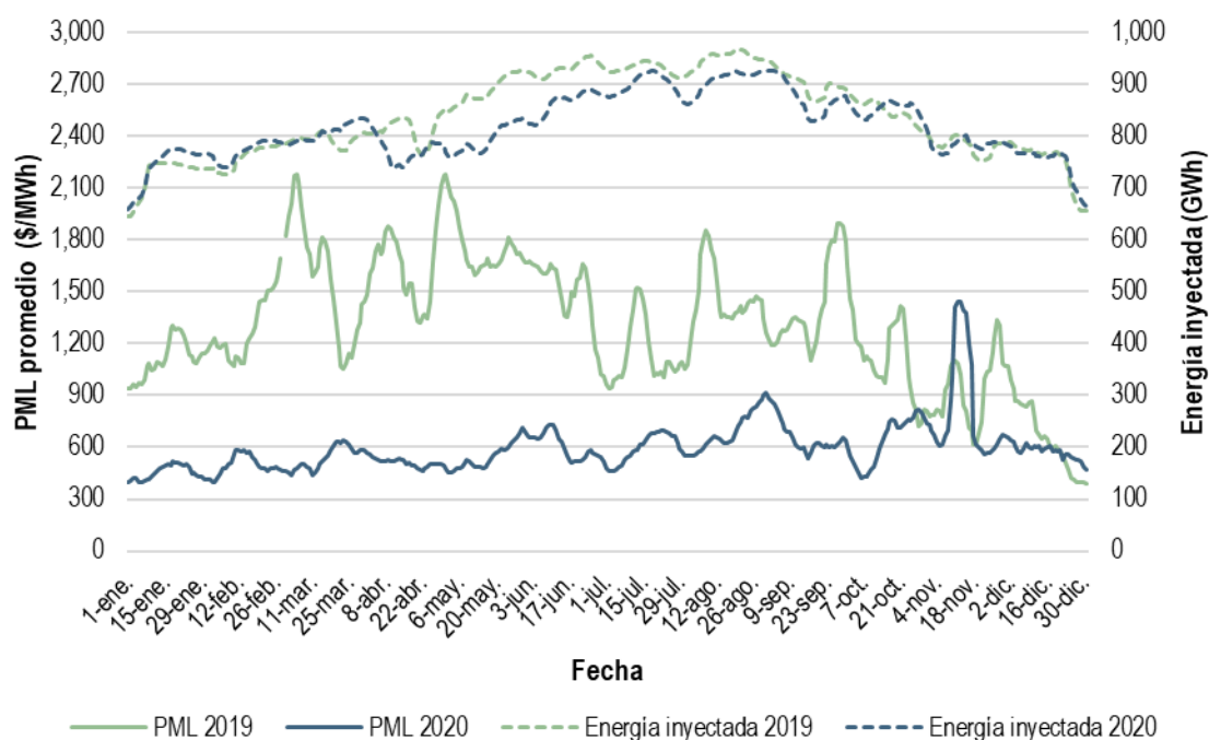
Gráfica 211. PML promedio y energía inyectada diarios en el MDA del SIN, 2019 y 2020
