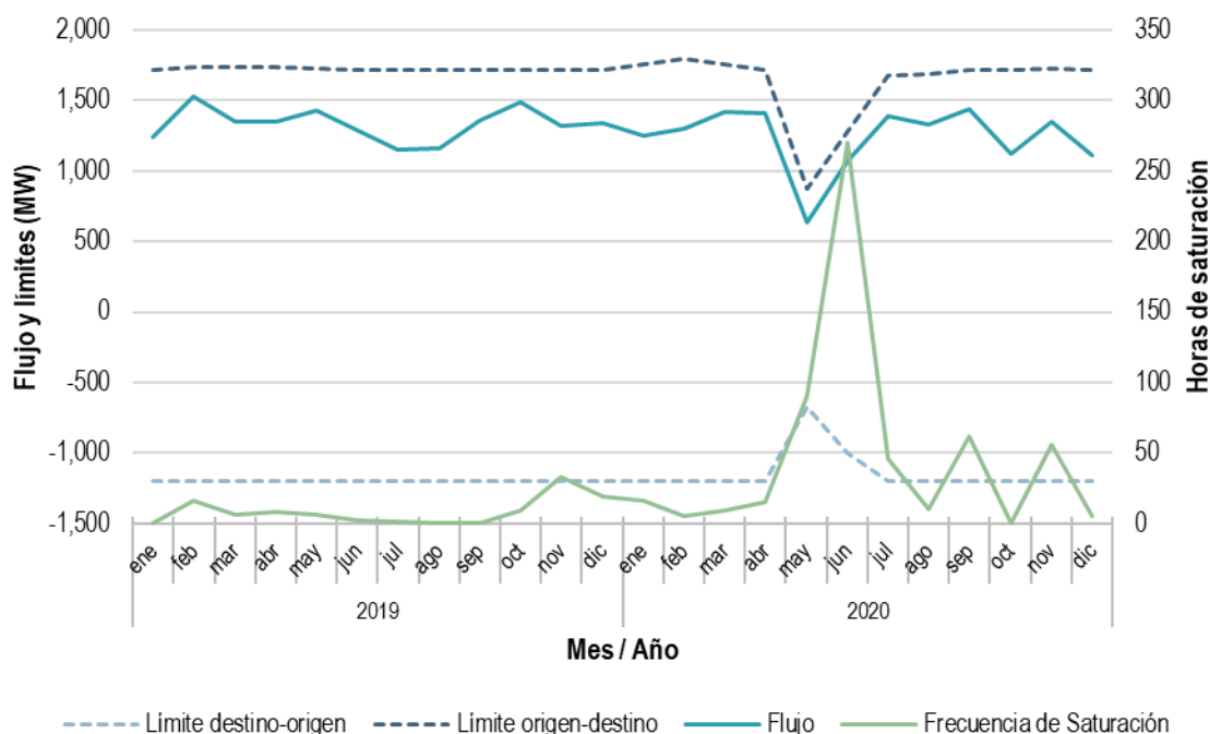
Gráfica 42. Flujo y límites de transmisión promedio horario por mes del enlace ORI-NES y su frecuencia de saturación mensual en el MDA, 2019 y 2020
