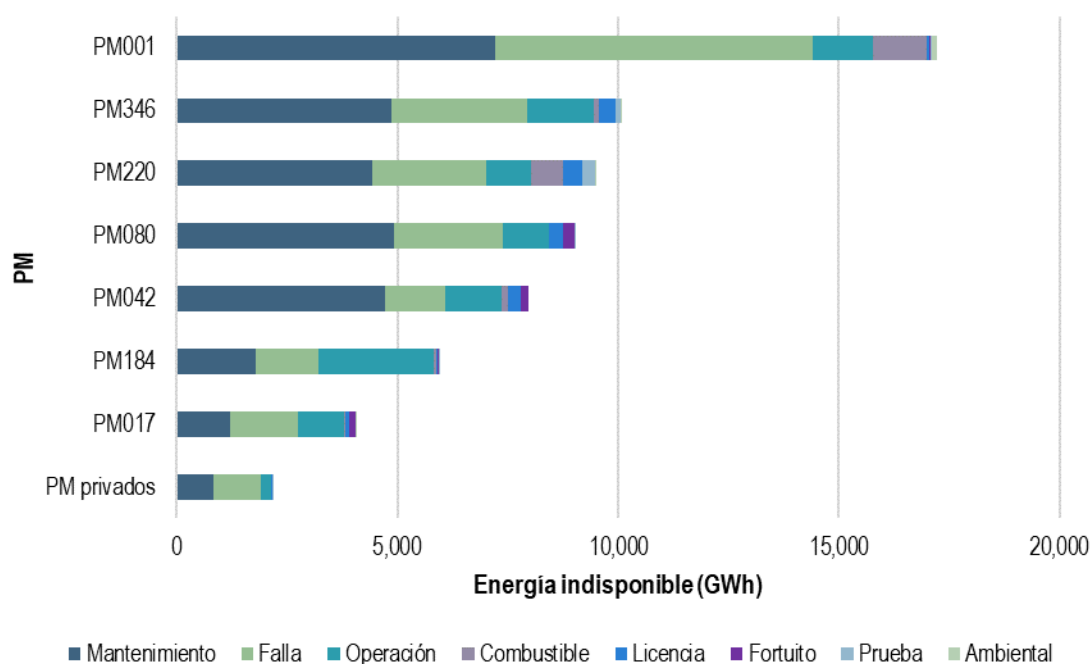
Gráfica 252. Energía indisponible por PM y tipo de salida de UCE, 2020
