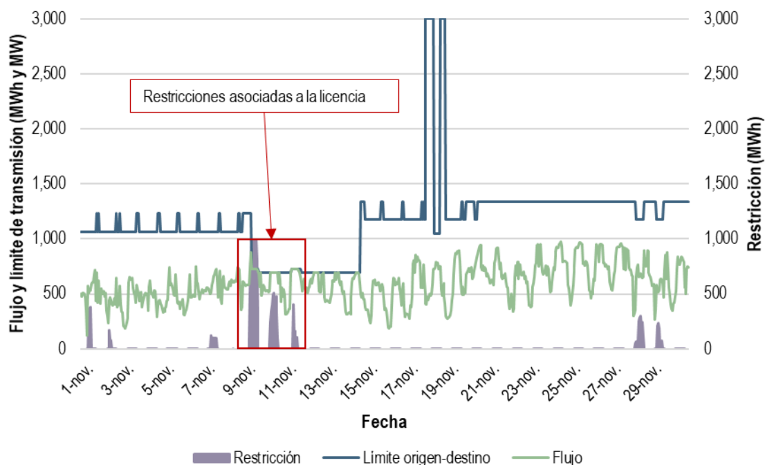
Gráfica 54. Flujo y límites de transmisión de la licencia en Sonora Sur- Sinaloa en el MDA, noviembre de 2020
