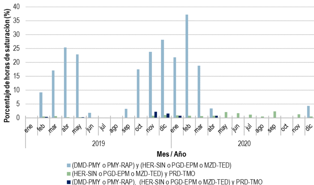
Gráfica 30. Saturación en el MDA de más de un enlace de las GCR NOR, NTE y NES, 2019 y 2020
