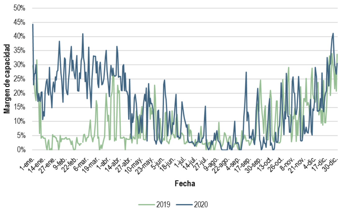
Gráfica 74. Margen de capacidad después de reservas en la hora de menor margen diario en el MDA del BCA, 2019 y 2020
