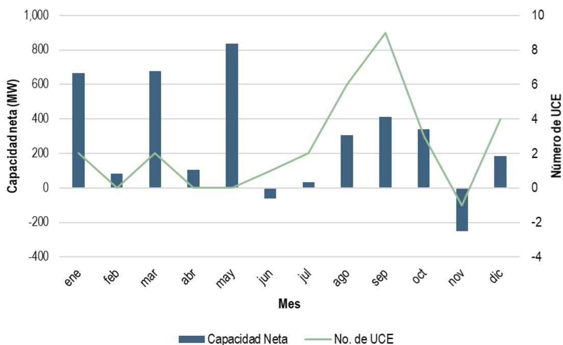
Gráfica 124. Cambio en la capacidad neta por altas y bajas y número de UCE del SEN por mes, 2020
