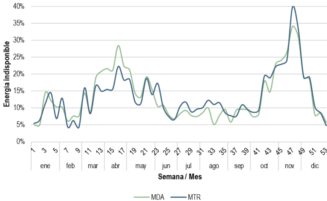
Gráfica 242. Energía indisponible reflejada en las Ofertas de Venta TE en el MDA y el MTR del BCA, 2020
