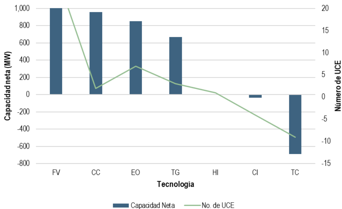
Gráfica 123. Cambio en la capacidad neta por altas y bajas y número de UCE del SEN por tecnología, 2020
