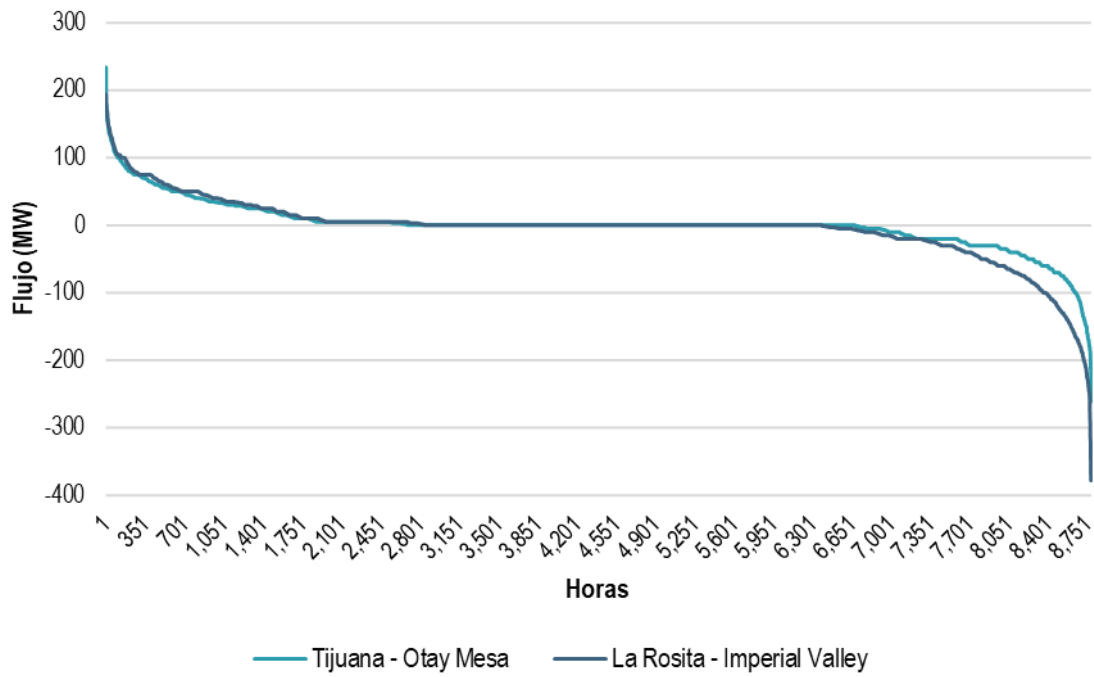
Gráfica 231. Curva de duración de flujos internacionales de energía en los Enlaces de Interconexión del BCA con el CAISO, 2020
