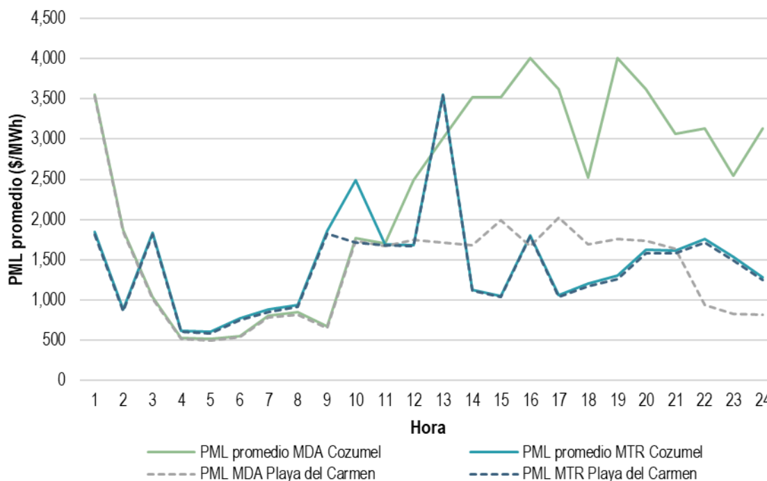
Gráfica 136. Diferencias en los PML promedio de la ZC de Cozumel entre el MDA y el MTR, 4 de marzo de 2020
