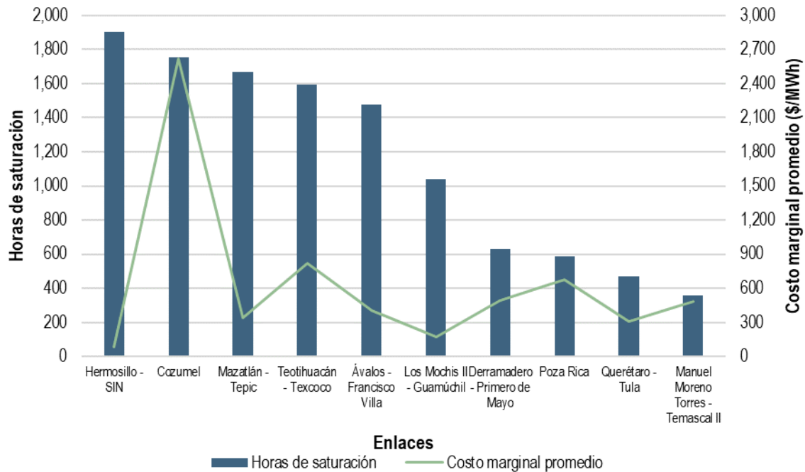
Gráfica 222. Horas de saturación y costo marginal promedio en los 10 Enlaces de Interconexión no fronterizos más congestionados en el MDA del SEN, 2020
