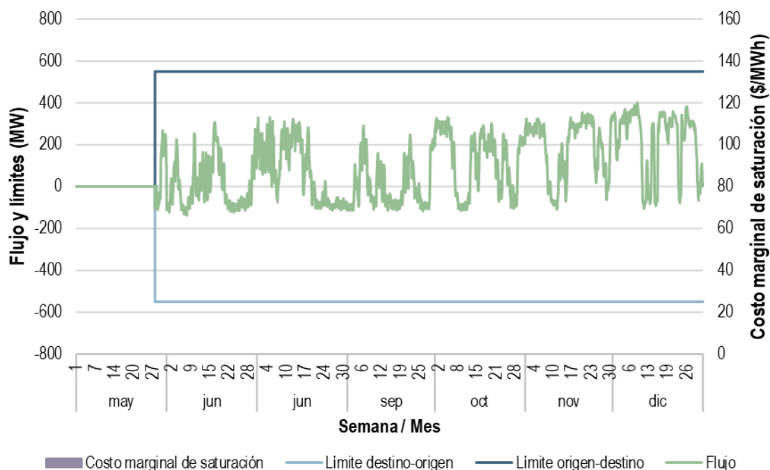
Gráfica 49. Límites de transmisión, flujo y costo marginal de saturación del enlace Matías Romero - Juile en el MDA, mayo a diciembre de 2020
