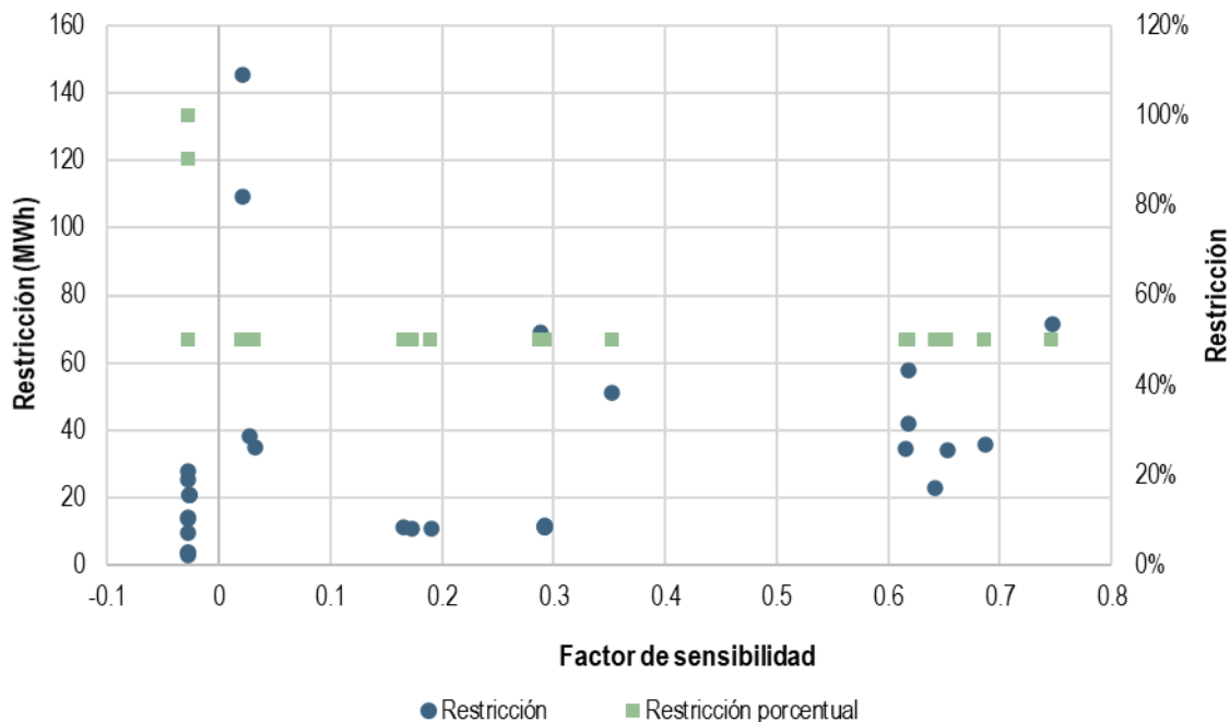
Gráfica 55. Restricciones a la generación de UCE RN en el MDA, según su factor de sensibilidad respecto a la licencia en Sonora Sur- Sinaloa, a la hora 15 del 9 de noviembre de 2020
