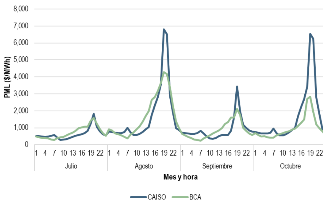
Gráfica 83. PML promedio en el CAISO y en el BCA (nodo 07IVY-230), julio a octubre de 2020
