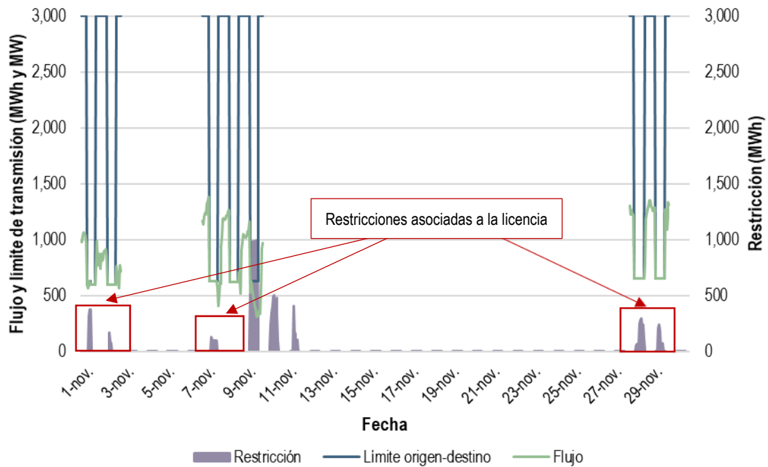
Gráfica 53. Flujo y límites de transmisión de la licencia Mazatlán-Tepic en el MDA, noviembre de 2020
