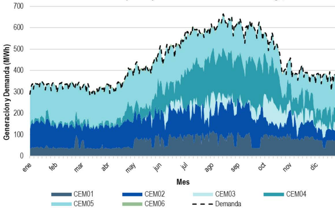
Gráfica 208. Generación por CE y demanda total en el Sistema Mulegé, 2020
