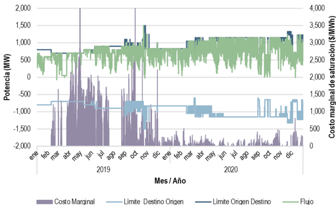
Gráfica 31. Límites de transmisión, flujo y costo marginal de saturación del enlace HER-SIN en el MDA, 2019 y 2020
