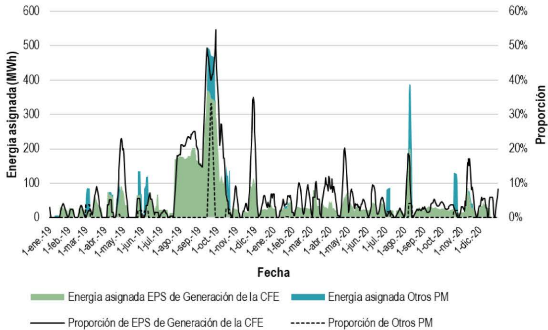
Gráfica 189. Energía asignada de las Ofertas de Venta TE asignables no despachables sobre el total de la energía térmica asignada en el BCA por grupo de PM, 2019-2020
