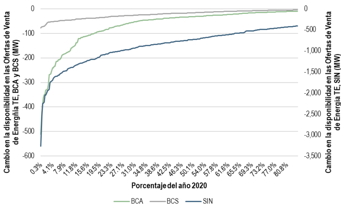
Gráfica 139. Estimación horaria de la indisponibilidad por falla en Tiempo Real por cambios en los LDEMáx de las Ofertas de Venta TE del MTR, 2020
