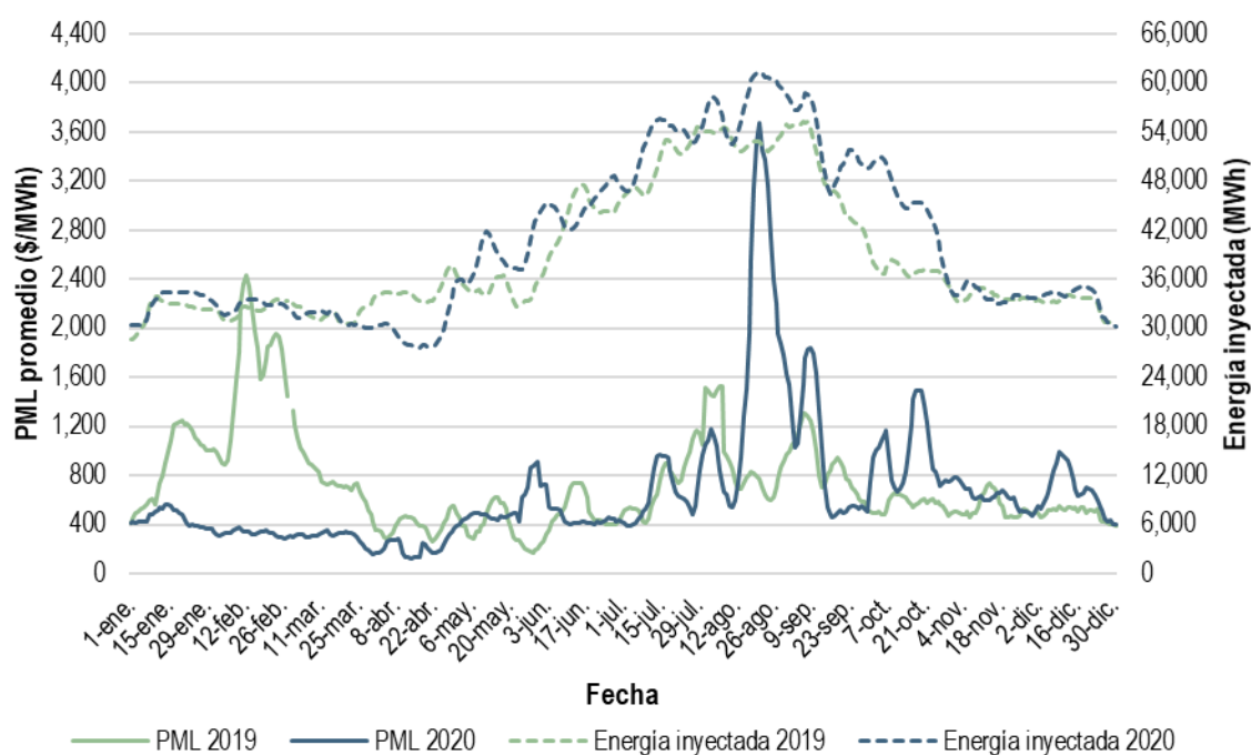
Gráfica 212. PML promedio y energía inyectada diarios en el MDA del BCA, 2019 y 2020
