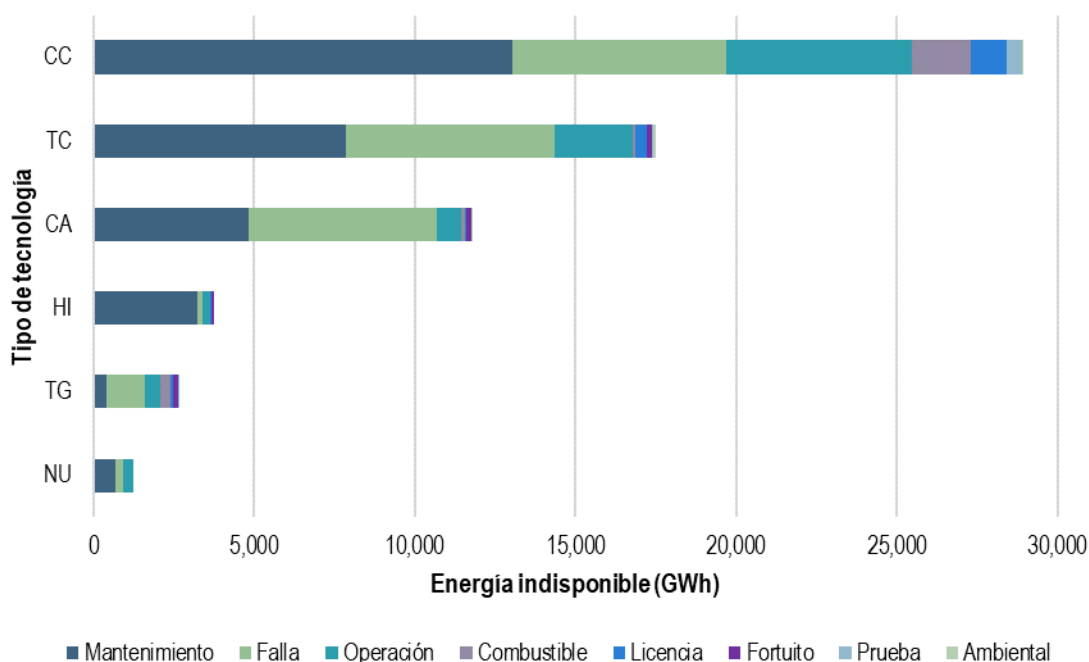
Gráfica 250. Energía indisponible por tipo de tecnología y tipo de salida de UCE, 2020 (1 de 2)
