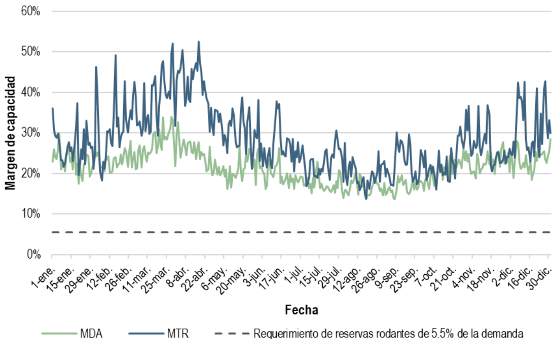
Gráfica 219. Margen de capacidad rodante promedio en el MDA y el MTR del BCA, 2020
