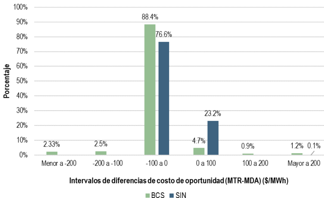
Gráfica 116. Diferencias de los costos de oportunidad de RR10 entre el MDA y el MTR del BCS y SIN, mayo a diciembre de 2020
