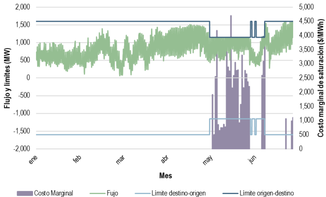
Gráfica 44. Límites de transmisión, flujo y costo marginal de saturación del enlace Malpaso – Tabasco en el MDA, enero a junio de 2020
