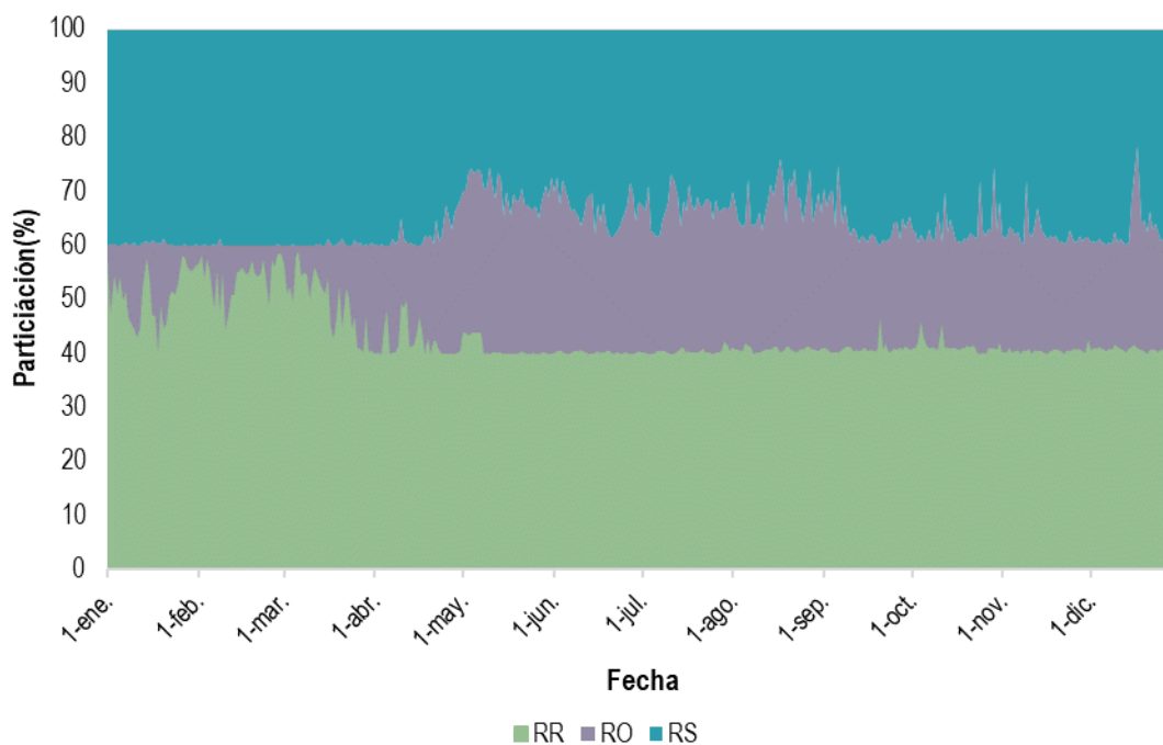
Gráfica 26. Participación de la asignación de las RR, RO y RS en el requerimiento de la RS, 2020
