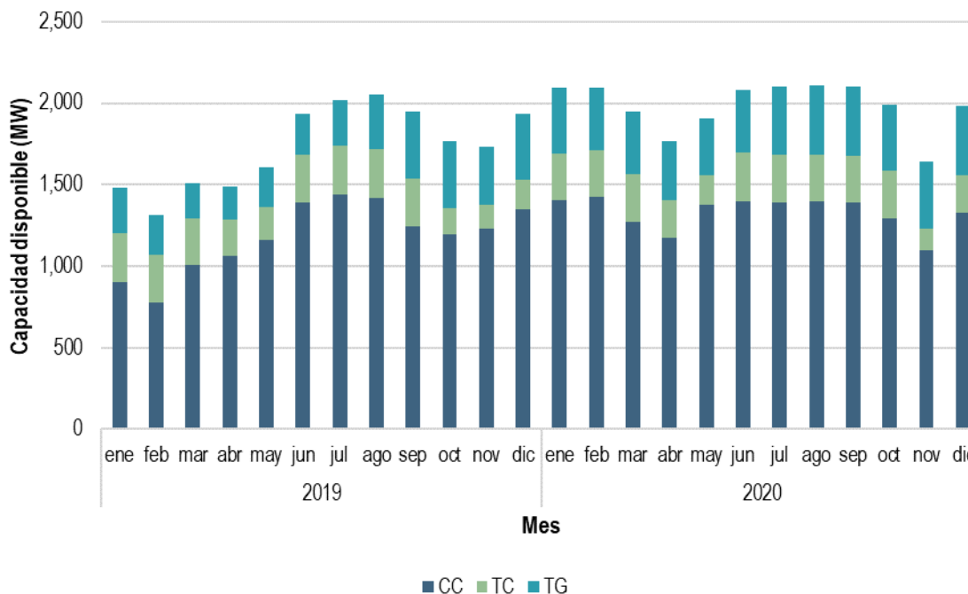
Gráfica 78. Capacidad disponible promedio horaria por tipo de tecnología de las Ofertas de Venta TE en el MDA en el BCA, 2019 y 2020
