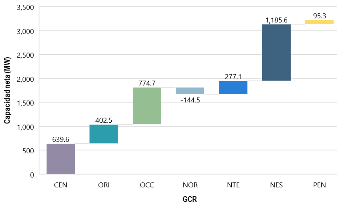
Gráfica 5. Capacidad neta adicional que se integró por GCR al SIN, 2020
