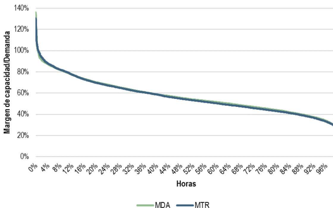
Gráfica 140. Curva de duración del margen de capacidad en el MDA y el MTR del SIN, 2020
