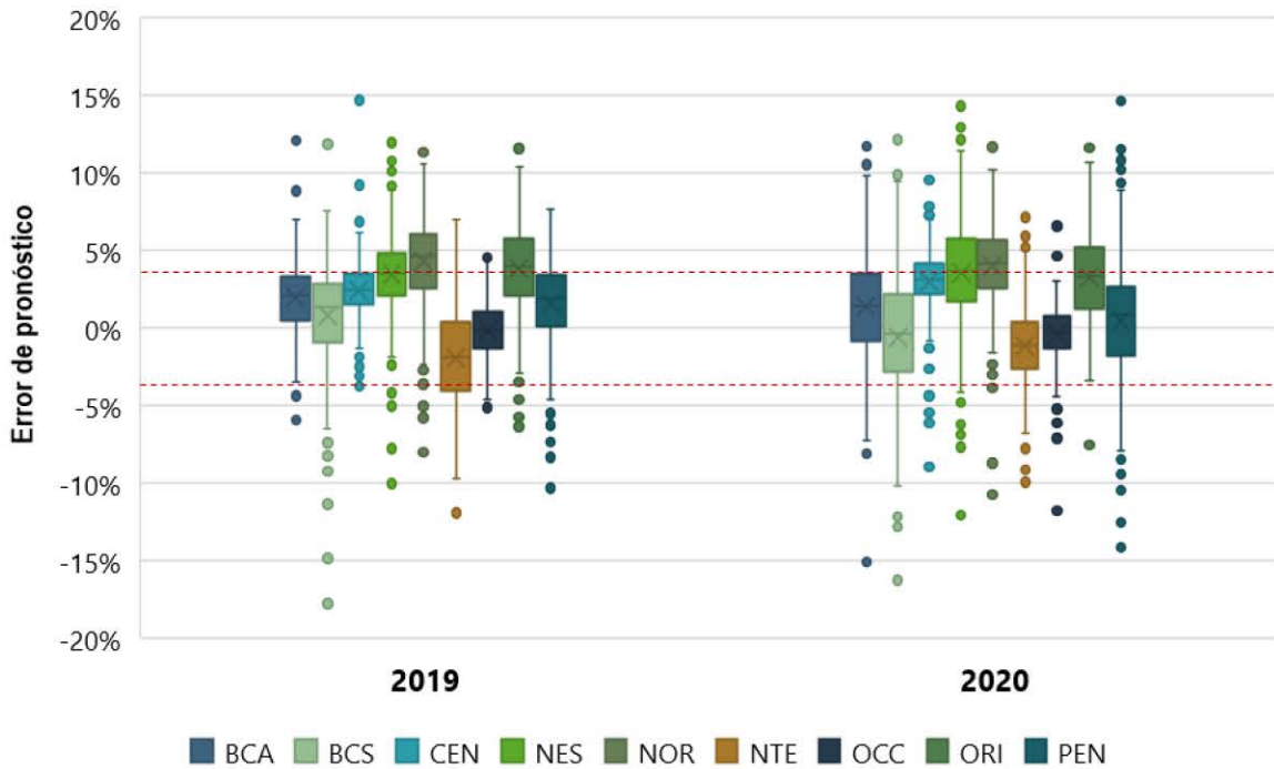
Gráfica 167. Distribución de los errores de pronóstico de carga por GCR, 2019 y 2020
