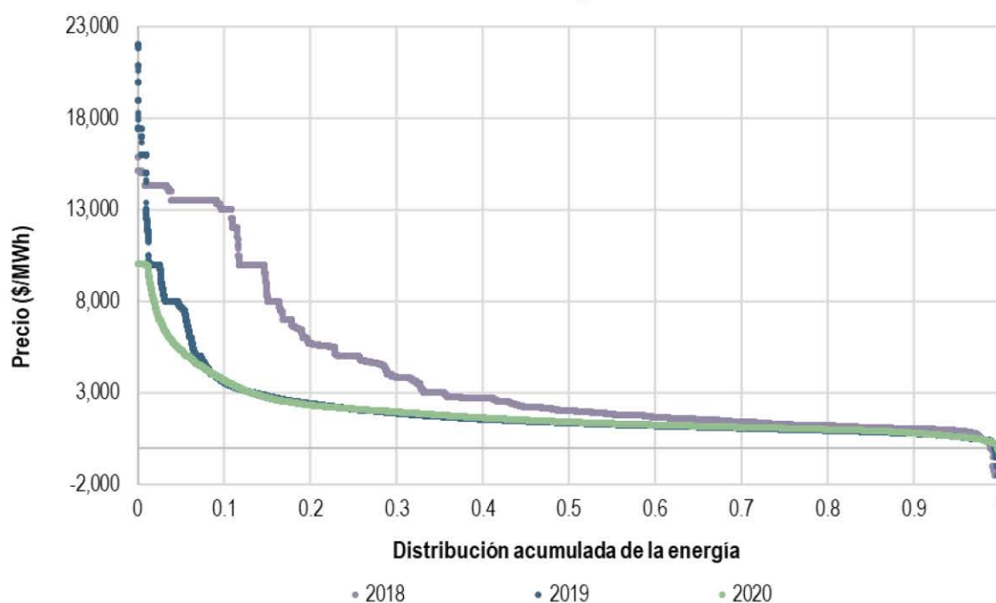
Gráfica 183. Curva de duración de las ofertas de importación en los nodos de transacciones internacionales del BCA, 2018, 2019 y 2020
