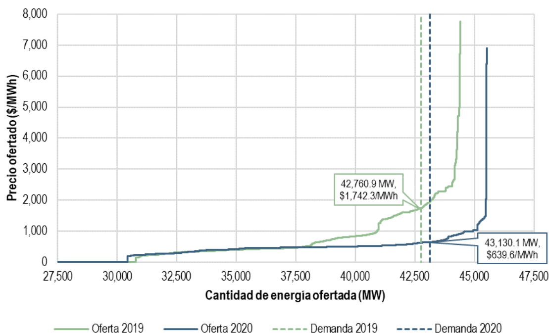
Gráfica 6. Curvas de oferta asignada y demanda, 12 de junio de 2019 y 26 de agosto de 2020 a la hora 17
